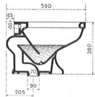
FF 3089. - Cuvette à action siphonique. Modèle non-contact.
