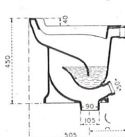
FF 3372. - Cuvette non-contact à chasse directe. Sortie arrière sous le socle. A = 200 mm.
