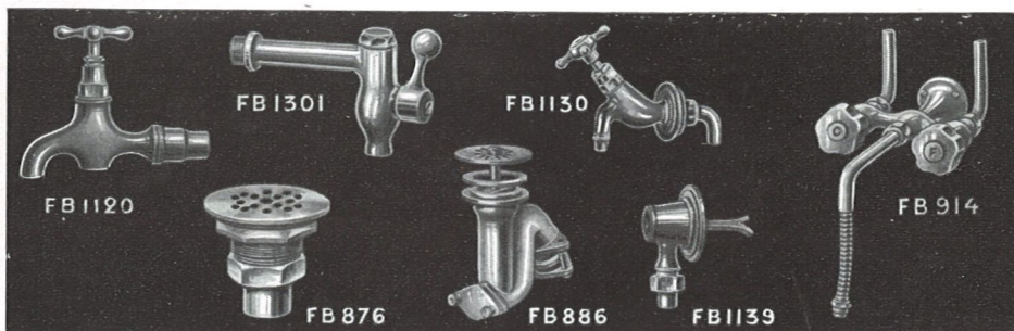
FB 1301. - Robinet d'évier à bascule avec dispositif anti-bélier.
