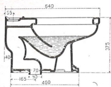
FF 3180. - Cuvette à action siphonique. Modèle spécial pour réservoir FF 4053.
