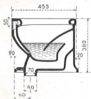
FF 3250. - Cuvette à action siphonique. Modèle à sortie arrière sous le socle.
