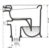
FF 3405. - Cuvette à fond plat. Modèle à sortie arrière sous le socle.
