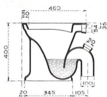
FF 3352. - Cuvette à chasse directe. Sortie verticale dans l'axe.
