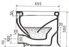
FF 3290. - Cuvette à action siphonique. Modèle à sortie arrière horizontale.
