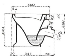
FF 3353. - Cuvette à chasse directe. Sortie oblique dans l'axe.
