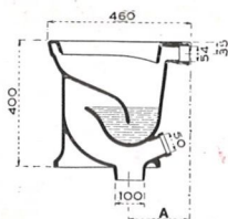
FF 3371. - Cuvette à chasse directe. Sortie arrière sous le socle. A = 195 mm.
