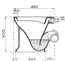
FF 3354. - Cuvette à chasse directe. Sortie oblique à droite.
