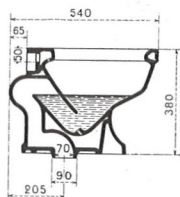
FF 3088. - Cuvette à action siphonique. Modèle oval.
