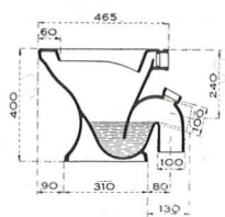
FF 3362. - Cuvette pour emploi sans abattant. Sortie verticale dans l'axe.
